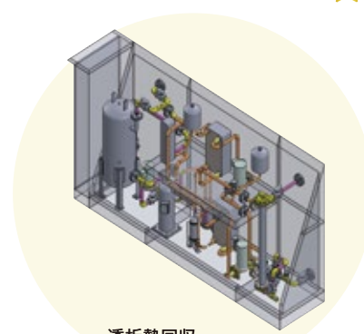
透析熱回収 ヒートポンプユニット内部
